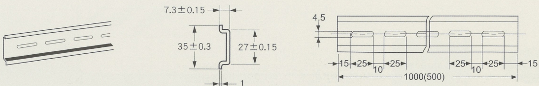
DIN導軌尺寸圖(參考)
